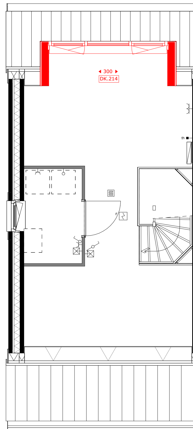
DK.214 = dakkapel achtergevel (breedte c.a. 3m)
