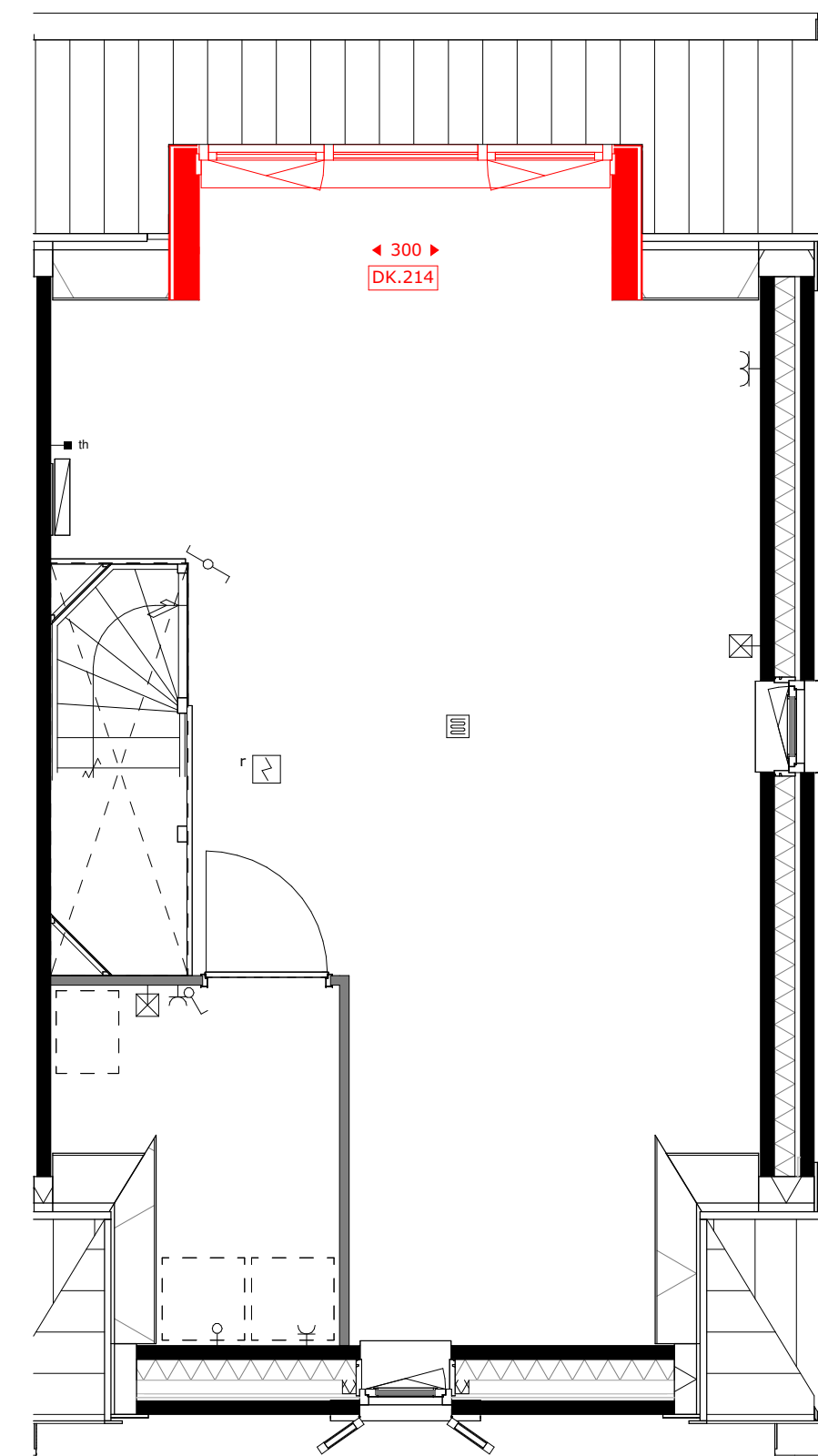
DK.214 = dakkapel achtergevel (breedte c.a. 3m)
